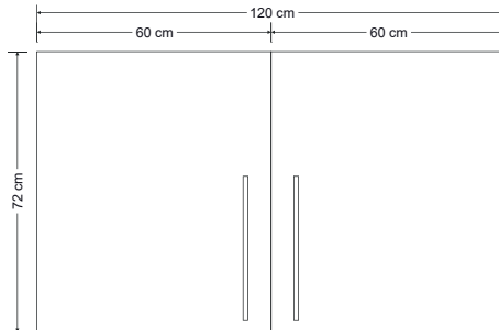
HS 120 - Croquis
