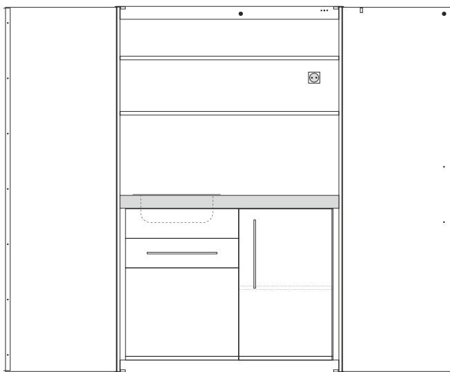
Croquis: SKM - Modelo básico sin aparatos
